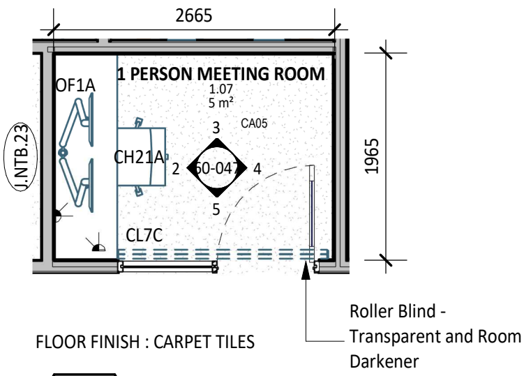
1 PLAN DETAIL 1 : 50
